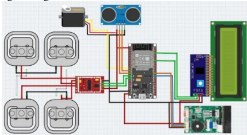
Gbr. 6 Perancangan Perangkat Keras
