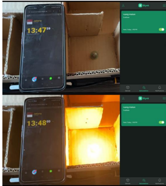
Gbr 17. Automation pada ruang makan
