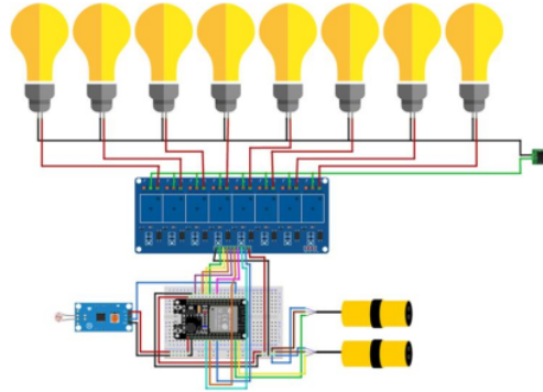
Gbr 10. Perancangan Perangkat Keras
