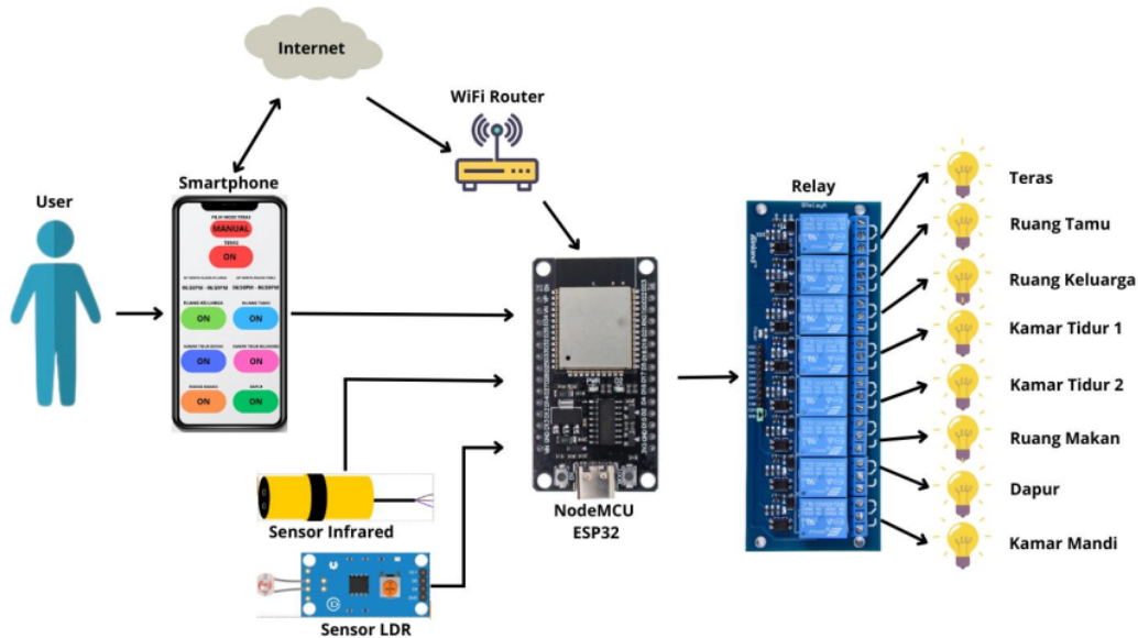
Gbr 6. Rancangan Sistem Kendali Otomatis
