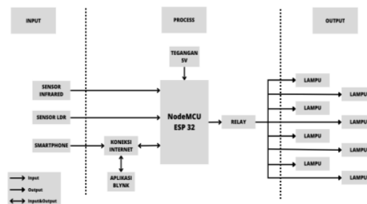
Gbr 8. Diagram Blok Sistem
