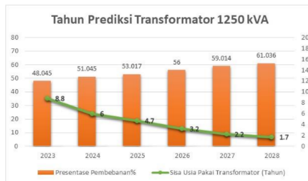
Gambar 2. Grafik Prediksi Usia Pakai Transformator 1250 KVA
