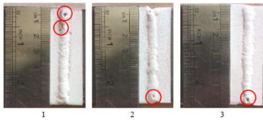
Gambar 12. Analisa Cacat Pengelasan Tungsten 1,6 mm Arus 100 A
