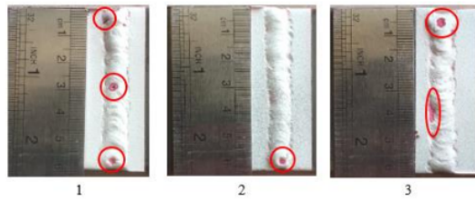
Gambar 16. Analisa Cacat Pengelasan Tungsten 2,4 mm Arus 100 A
