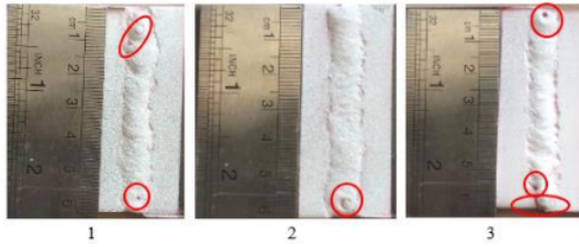
Gambar 18. Analisa Cacat Pengelasan Tungsten 3,2 mm Arus 100 A
