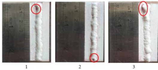
Gambar 13. Analisa Cacat Pengelasan Tungsten 1,6 mm Arus 120 A
