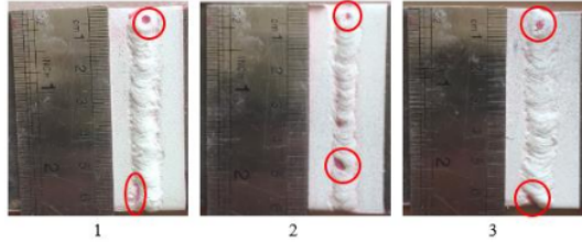
Gambar 11. Analisa Cacat Pengelasan Tungsten 1,6 mm Arus 80 A
