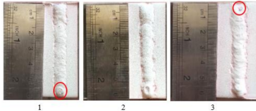
Gambar 19. Analisa Cacat Pengelasan Tungsten 3,2 mm Arus 120 A
