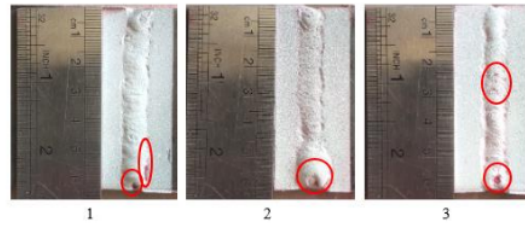
Gambar 15. Analisa Cacat Pengelasan Tungsten 2,4 mm Arus 100 A
