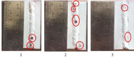
Gambar 17. Analisa Cacat Pengelasan Tungsten 3,2 mm Arus 80 A
