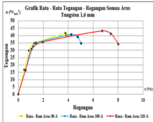
Gambar 22. Grafik Rata-Rata Tegangan – Regangan Tungsten 1,6 mm Arus 80 A, 100 A, 120 A
