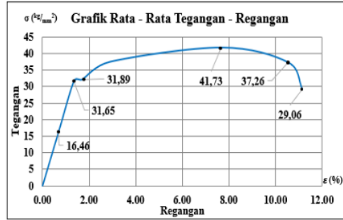
Gambar 21. Grafik Rata – Rata Tegangan – Regangan Raw Material
