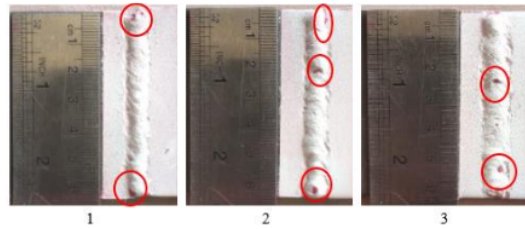
Gambar 14. Analisa Cacat Pengelasan Tungsten 2,4 mm Arus 80 A
