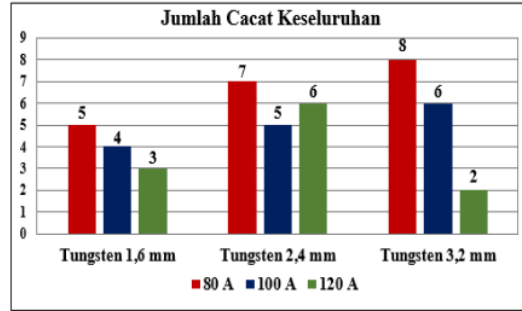
Gambar 20. Diagram Jumlah Cacat Keseluruhan
