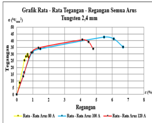
Gambar 23. Grafik Rata-Rata Tegangan – Regangan Tungsten 2,4 mm Arus 80 A, 100 A, 120 A
