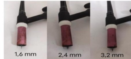
Gambar 2. Variasi Diameter Tungsten
