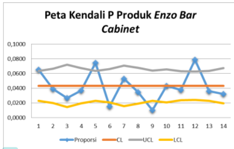
Gambar 4, Peta Kendali Cacat Produk
