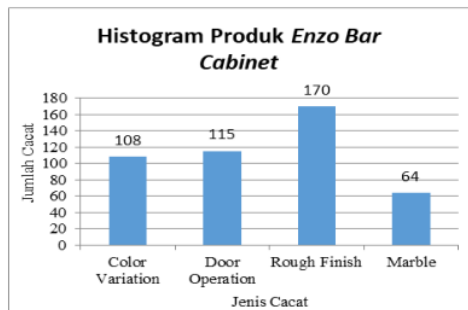
Gambar 2, Histogram Produk Enzo Bar Cabinet
