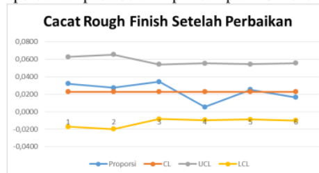
Gambar 13, Peta Kendali P Setelah Perbaikan
