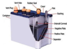
Gambar 2 baterai
