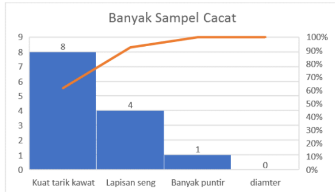
Gambar 5. Diagram pareto jumlah cacat
