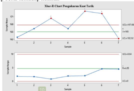
Gambar 6. Peta Kendali X-bar Dan R Kuat Tarik
