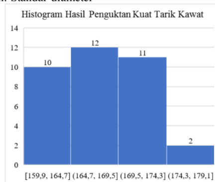
Gambar 2. Histogram hasil pengukuran kuat tarik
