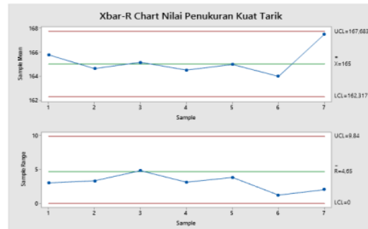
Gambar 15 Peta Kendali X-bar R nilai uji kuat tarik setelah perbaikan
