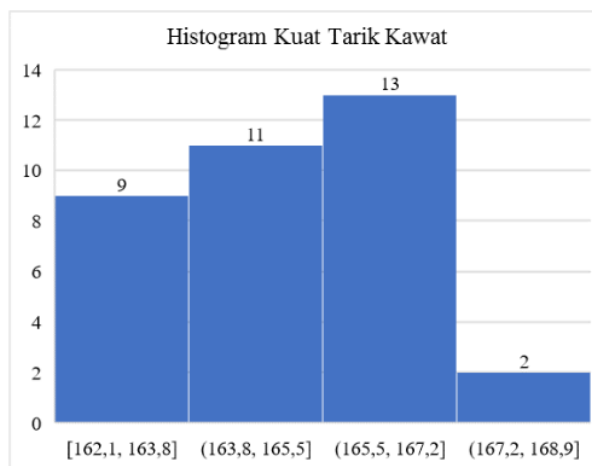
Gambar 14. Histogram hasil uji kau tarik setelah perbaikan
