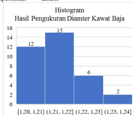
Gambar 1. Histogram pengukuran diameter
