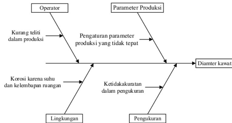
Gambar 13. Diagram sebab akibat diameter kawat
