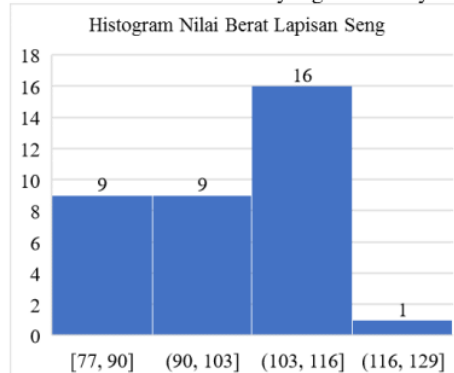
Gambar 4. Histogram hasil pengukuran berat seng
