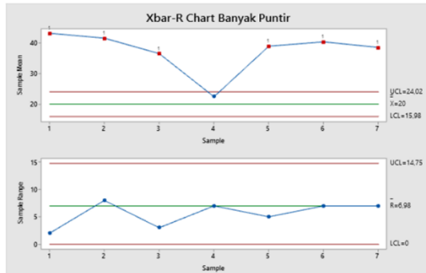
Gambar 7. Peta kendali X-bar R nilai banyak puntir
