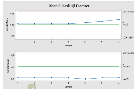
Gambar 9. Peta kendali X-bar R hasil pengukuran diameter
