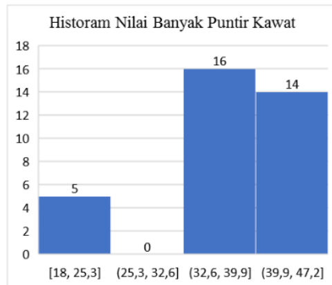
Gambar 3. Histogram hasil pengukuran puntir kawat
