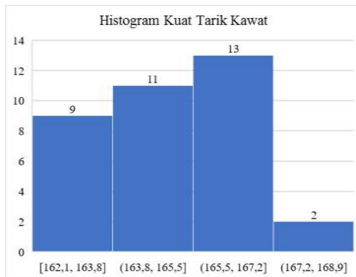
Gambar 14. Histogram hasil uji kau tarik setelah perbaikan
