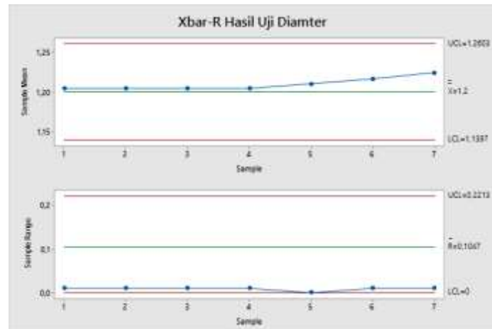
Gambar 9. Peta kendali X-bar R hasil pengukuran diameter
