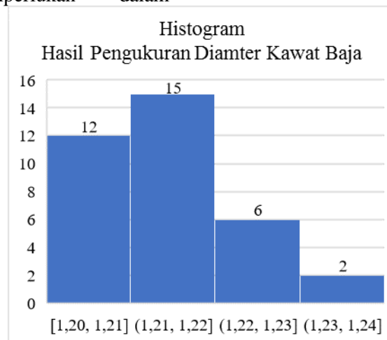
Gambar 1. Histogram pengukuran diameter
