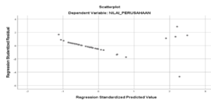
Gambar 4.3 Uji Heteroskedasitas
