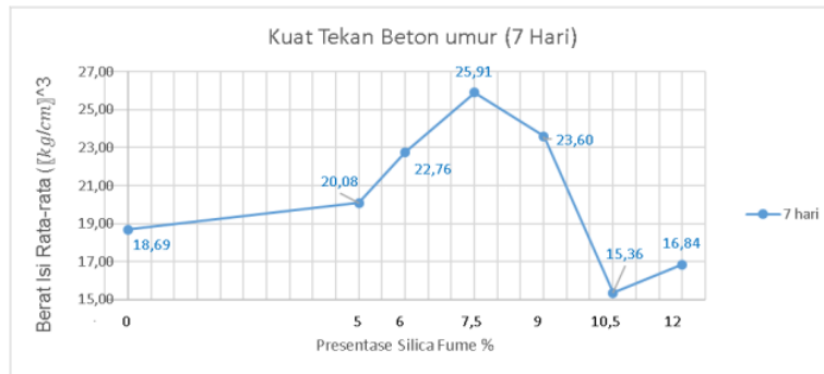
Gambar 2 Grafik Kuat Tekan Beton Umur 7 hari
