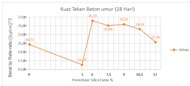
Gambar 3 Grafik Kuat Tekan Beton Umur 28 hari
