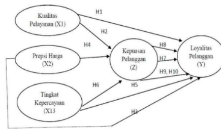
GAMBAR 2.1 KERANGKA KONSEPTUAL
