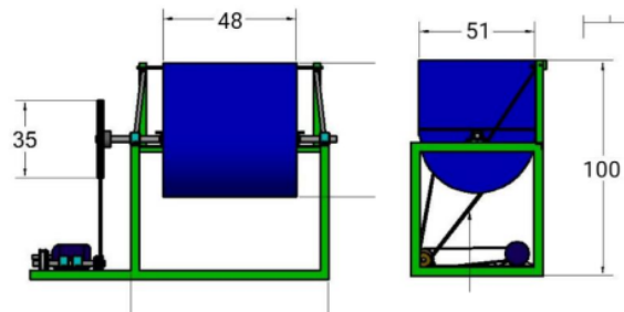
Gambar 2. Desain Ukuran Alat
