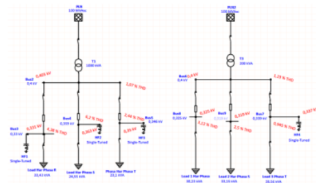
Gambar 3. Simulasi SLD dengan Filter
