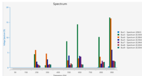
Gambar 5. Spektrum Harmonisa tanpa Filter
