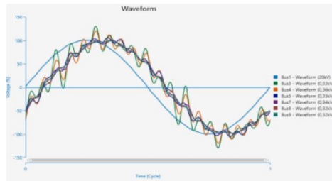
Gambar 4. Gelombang Harmonisa tanpa Filter
