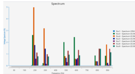
Gambar 7. Spektrum Harmonisa dengan Filter
