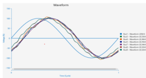
Gambar 6. Gelombang Harmonisa dengan Filter
