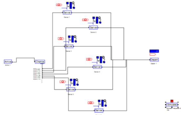
Gambar 4. 7 Skenario perbaikan penambahan server ke-6
