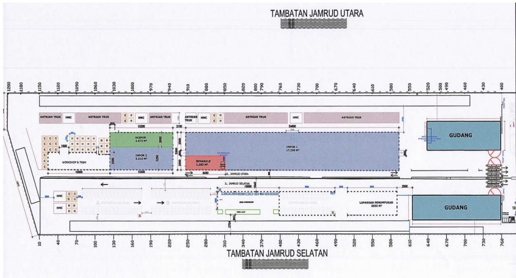
Lampiran 1. 2 Layout PT Pelindo (Persero) cabang Tanjung Perak, divisi Terminal Jamrud
