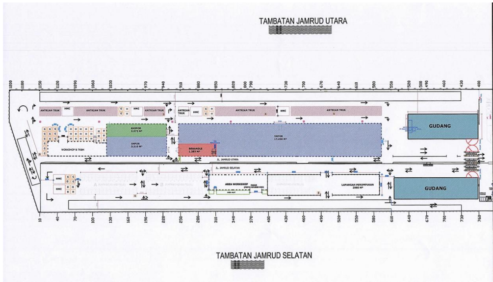
Lampiran 1. 3 Arah lalu lintas PT Pelindo (Persero) cabang Tanjung Perak, divisi Terminal Jamrud
