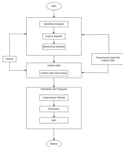
Gambar 1. Kerangka Pemikiran
