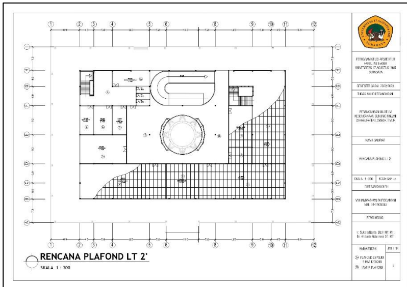
Lampiran 6 rencana plafond lt 2
