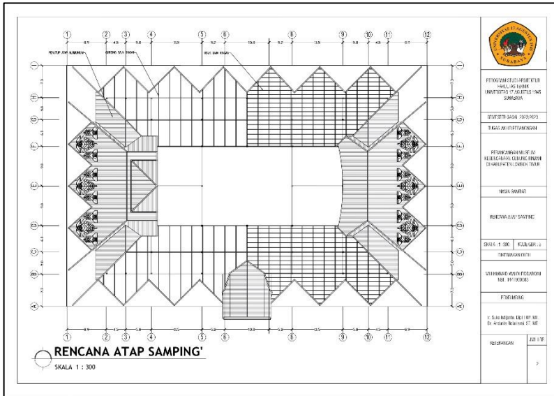
Lampiran 7 rencana atap samping Sumber : Analisis, 2023
