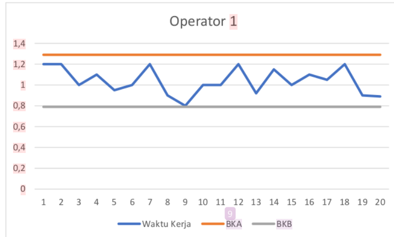
Gambar 4.1 Grafik Uji Keseragaman data Operator 1
