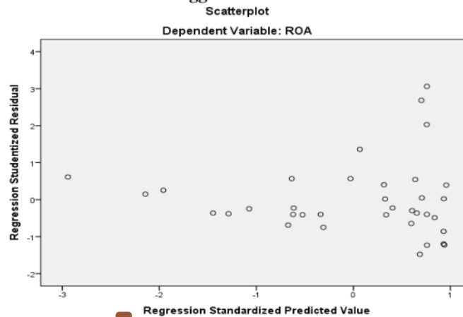
Gambar 1 Hasil Uji Heteroskedastisitas Menggunakan Variabel ROA
