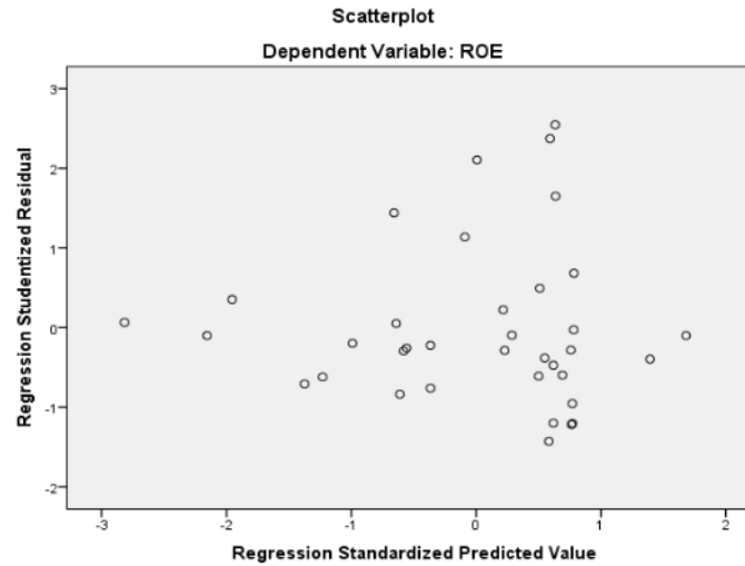
Gambar 2 Hasil Uji Heteroskedastisitas Menggunakan Variabel ROE
