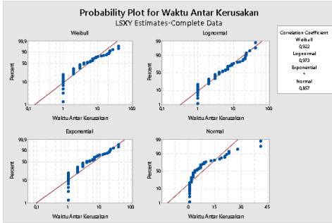
Lampiran 1 Hasil uji distribusi dan parameter data TTF & TTR komponen cutter.
