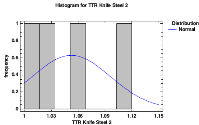
Gambar 4. Grafik Histogram Waktu Perbaikan Komponen Knife Steel 2
