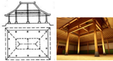
Gambar 13. Limisan Trajumas Lawakan & Soko Guru
