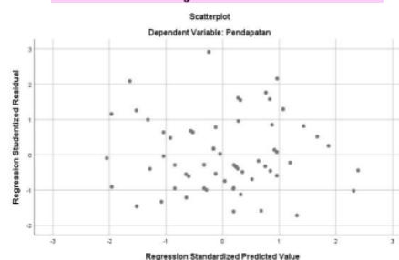
14 Gambar 4.2 Uji Heteroskedastisitas
