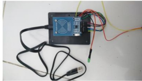
Gambar 4. 2 Alat RFID Reader
