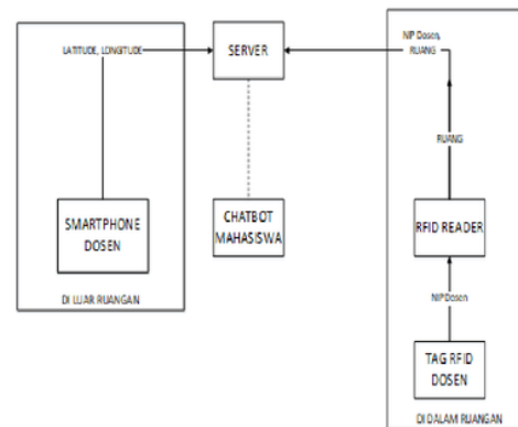
Gambar 3. 1 Blok diagram sistem
