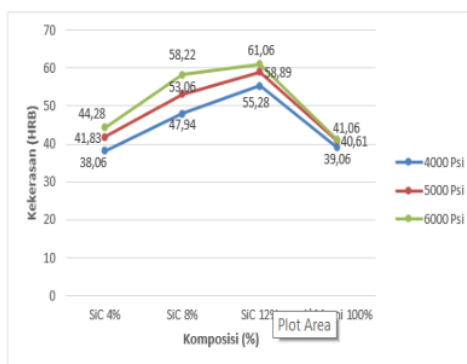
Grafik hubungan penambahan SiC & Al 100% kepada kekerasan
