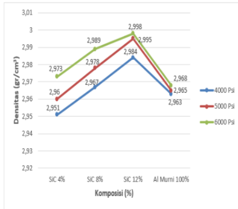
Grafik hubungan penambahan SiC & Al 100% kepada densitas
