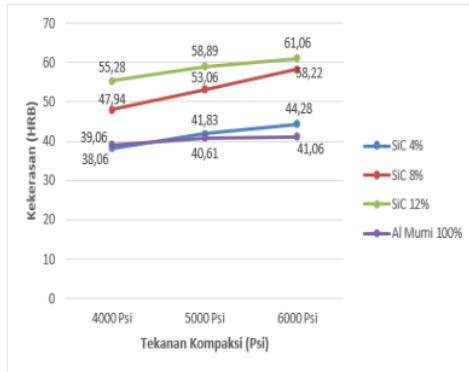
Grafik hubungan pematatan kepada kekerasan Al-SiC & Al 100%
