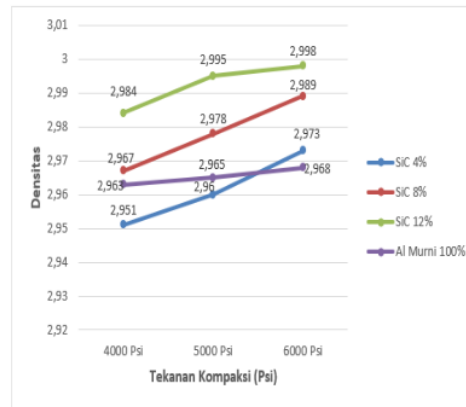
Grafik hubungan pemadatan kepada densitas Al-SiC & Al 100%
