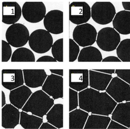
Gambar 1. Tahapan Proses Sintering
