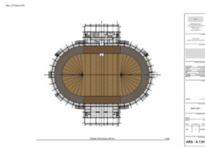
Gambar 6. Lantai 1 (sumber : penulis, 2023)
