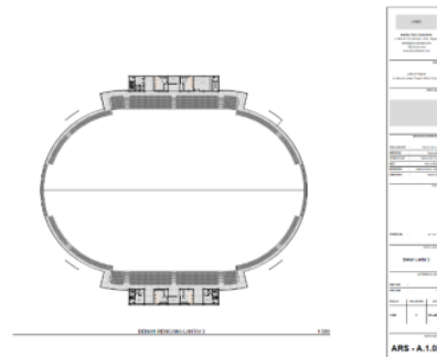
Gambar 8. Lantai 3 (sumber : penulis, 2023)
