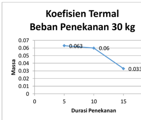
Gambar 9. Grafik rata-rata pengujian TGA
