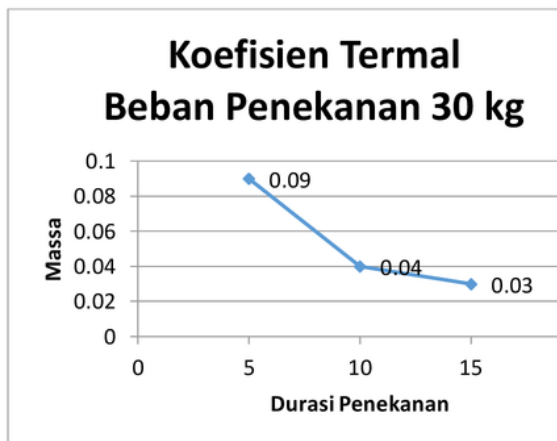
Gambar 6. Grafik rata-rata Pengujian TGA
