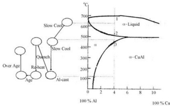
8 Gambar 3. Diagram fasa perubahan mikrostruktur paduan Al-Cu.
