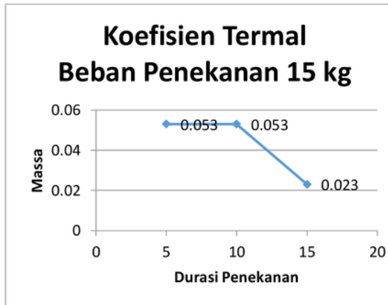
Gambar 8. Grafik rata-rata pengujian TGA
