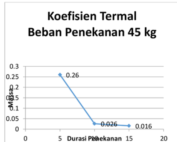
Gambar 7. Grafik rata-rata pengujian TGA
