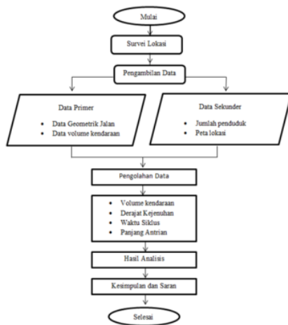
Gambar 1 Diagram Alir
