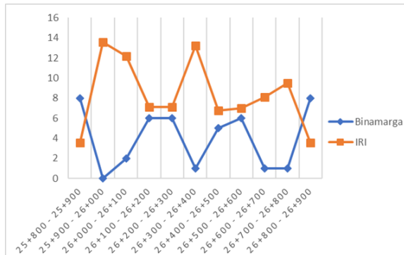
Gambar 4. Perbandingan Nilai Kerusakan Pada Ruas Jalan Gresik-Lamongan (Arah Lamongan)
