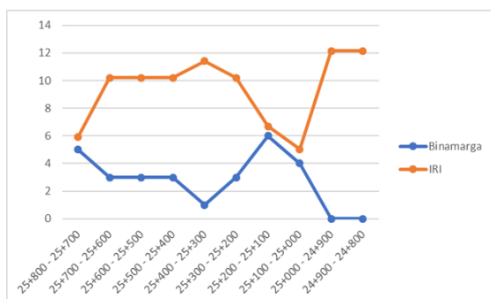
Gambar 6. Perbandingan Nilai Kerusakan Pada Ruas Jalan Raya Duduk Sampeyan (Arah Surabaya)
