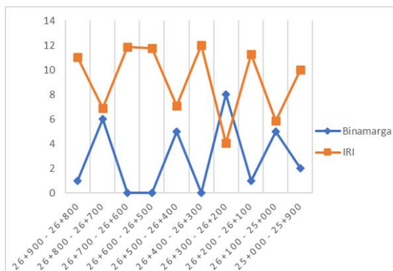
Gambar 5. Perbandingan Nilai Kerusakan Pada Ruas Jalan Raya Duduk Sampeyan (Arah Surabaya)
