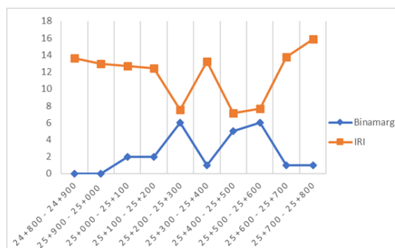
Gambar 3. Perbandingan Nilai Kerusakan Pada Ruas Jalan Gresik-Lamongan (Arah Lamongan)
