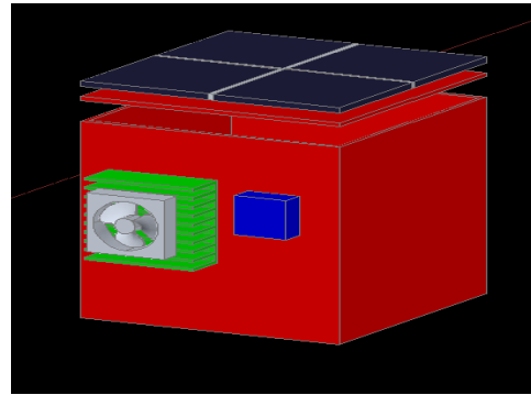
Gambar 7. Desain alat Pendingin Ikan Pengambilan Data
