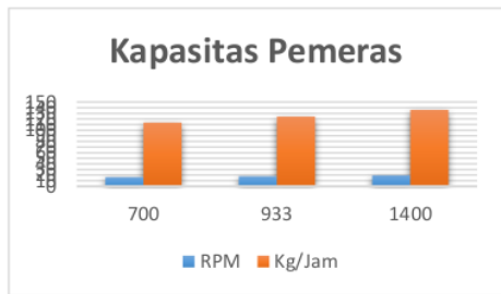
Gambar 4.2 Rekapitulasi hasil kapasitas pemas santan
