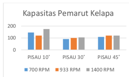
Gambar 4.1 Rekapitulasi hasil kapasitas pamarut kelapa
