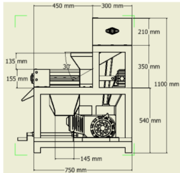
Gambar 6.1 desain pandangan samping
