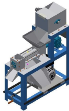
Gambar 6.4 Desain rancang bangun
