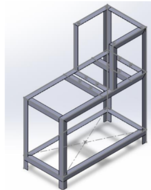
Gambar 6.5 Kerangka produk
