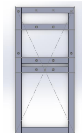
Gambar 6.6 rangka pandangan atas
