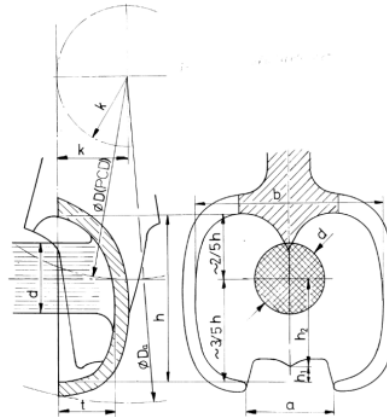
2 Gambar 1. Keterangan dimensi dari sudu pada turbin pelton (Eisenring, 1991)
