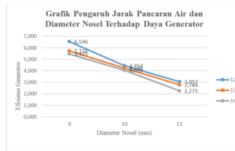
Gambar 10. Grafik pengaruh jarak pancaran air dan diameter nosel terhadap daya generator
