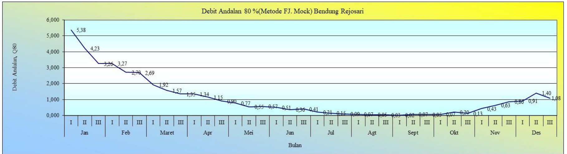
Gambar 4.8 Debit Andalan 80 %(Metode FJ. Mock) Bendung Rejosari Sumber : Hasil Analisis, 2023
