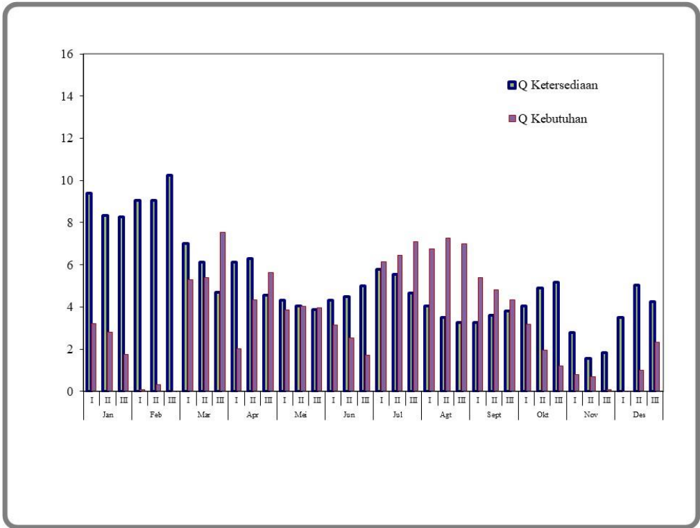
Gambar 4.9 Grafik Neraca Air Daerah Irigasi Bendung Rejosari Sumber : Hasil Analisis, 2023
