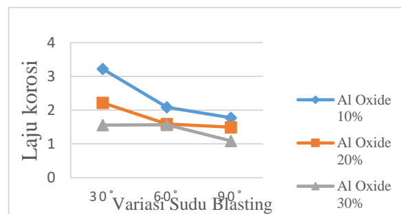
Gambar 4. 4 Grafik Hasil Pengujian Laju Korosi Spesimen A1, A2, A3, B1, B2, B3, C1, C2, C3 Perendaman Larutan HCl Selama 15 Hari.
