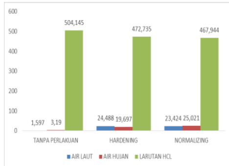
Gambar 4.4 Grafik Rata-rata laju percepatan (Mpy) specimen Baja ST 42 Tanpa Perlakuan Panas Dan Perlakuan Panas
