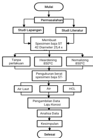
Gambar 1. skema pengujian perlakuan panas
