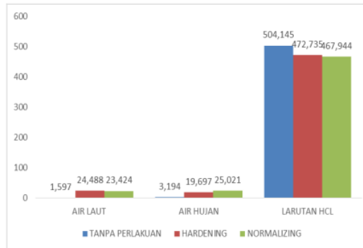
Gambar 5. Grafik Perbandingan laju korosi (mpy) Baja ST 42 Dengan Media Korosi.
