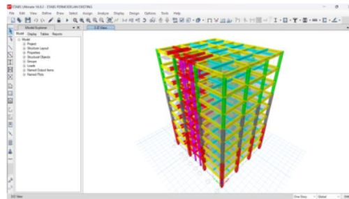
Gambar 6 permodelan Etabs kondisi existing
