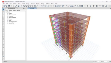
Gambar 8 permodelan Etabs kondisi modifikasi
