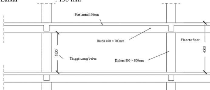
Gambar 4 potongan bangunan existing
