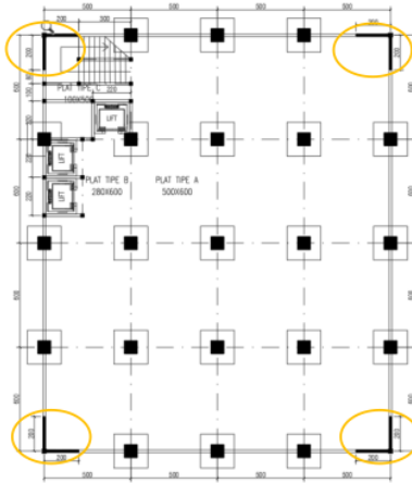
Gambar 5 denah bangunan modifikasi
