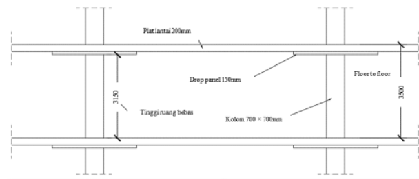
Gambar 7 potongan bangunan kondisi modifikasi
