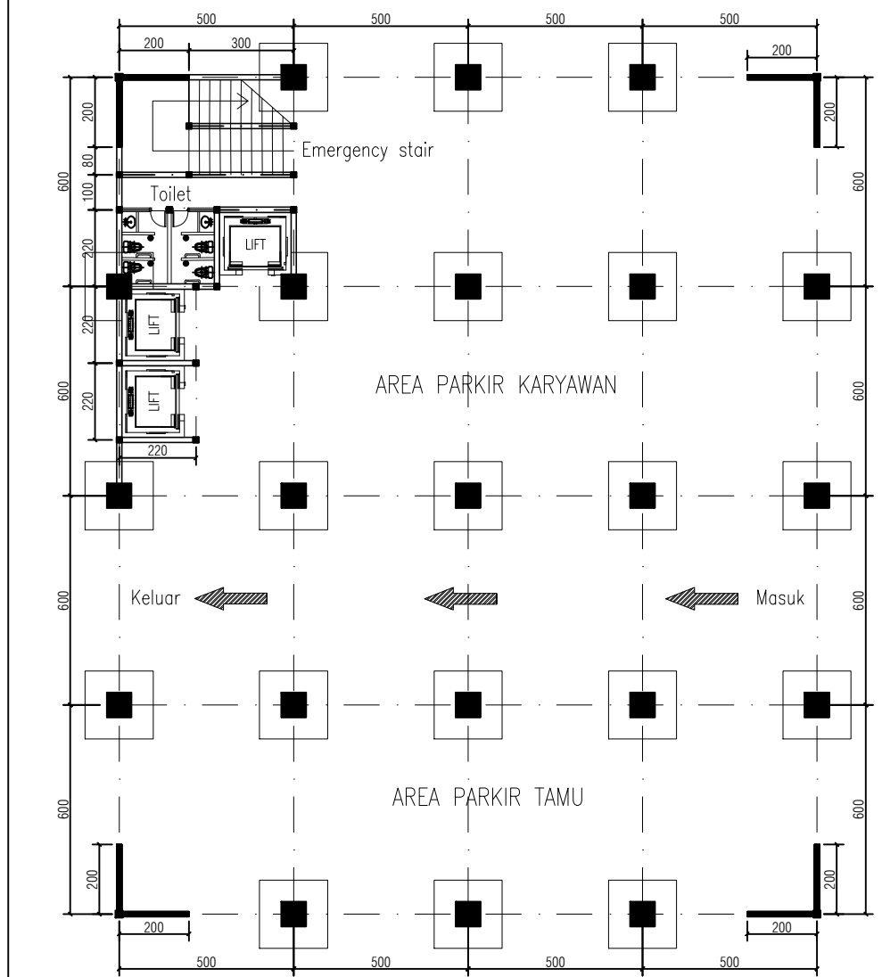
DENAH LANTAI DASAR SKALA 1 : 1
