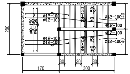
DET. TUL. TANGGA SKALA 1 : 1
