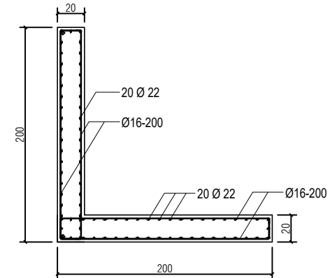
DET. TULANGAN SHEARWALL SKALA 1 : 1
