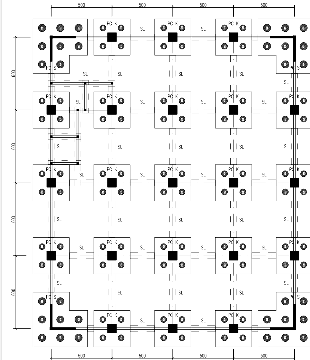
DENAH PONDASI SKALA 1 : 1
