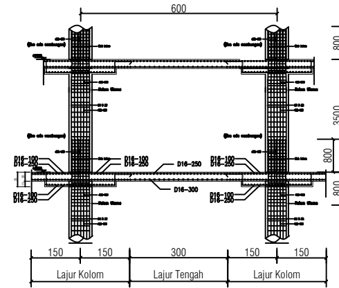
DET. KOLOM DAN FLAT SLAB SKALA 1 : 1
