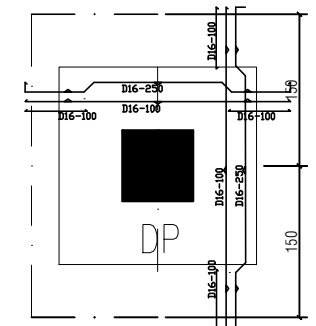
DET. TUL. DROP PANEL DAN FLAT SLAB SKALA 1 : 1
