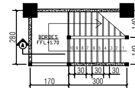
DENAH TANGGA SKALA 1 : 1
