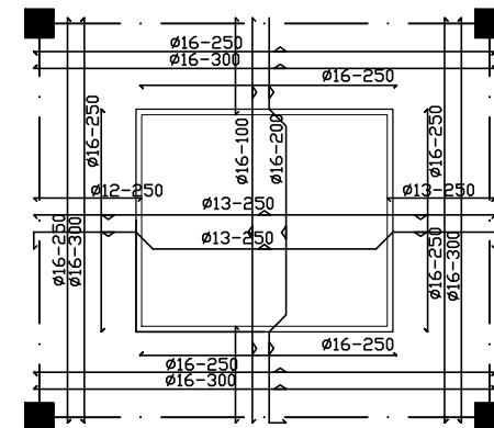
DET. TUL. FLAT SLAB SKALA 1 : 1
