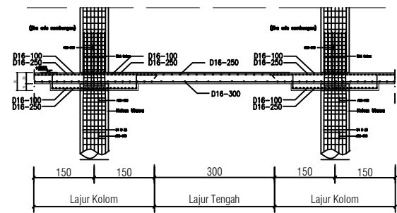
POTONAGAN FLAT SLAB DAN DROP PANEL SKALA 1 : 1
