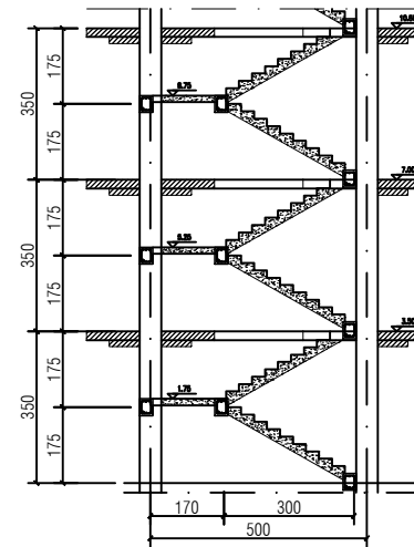
TAMPAK DEPAN TANGGA SKALA 1 : 1
