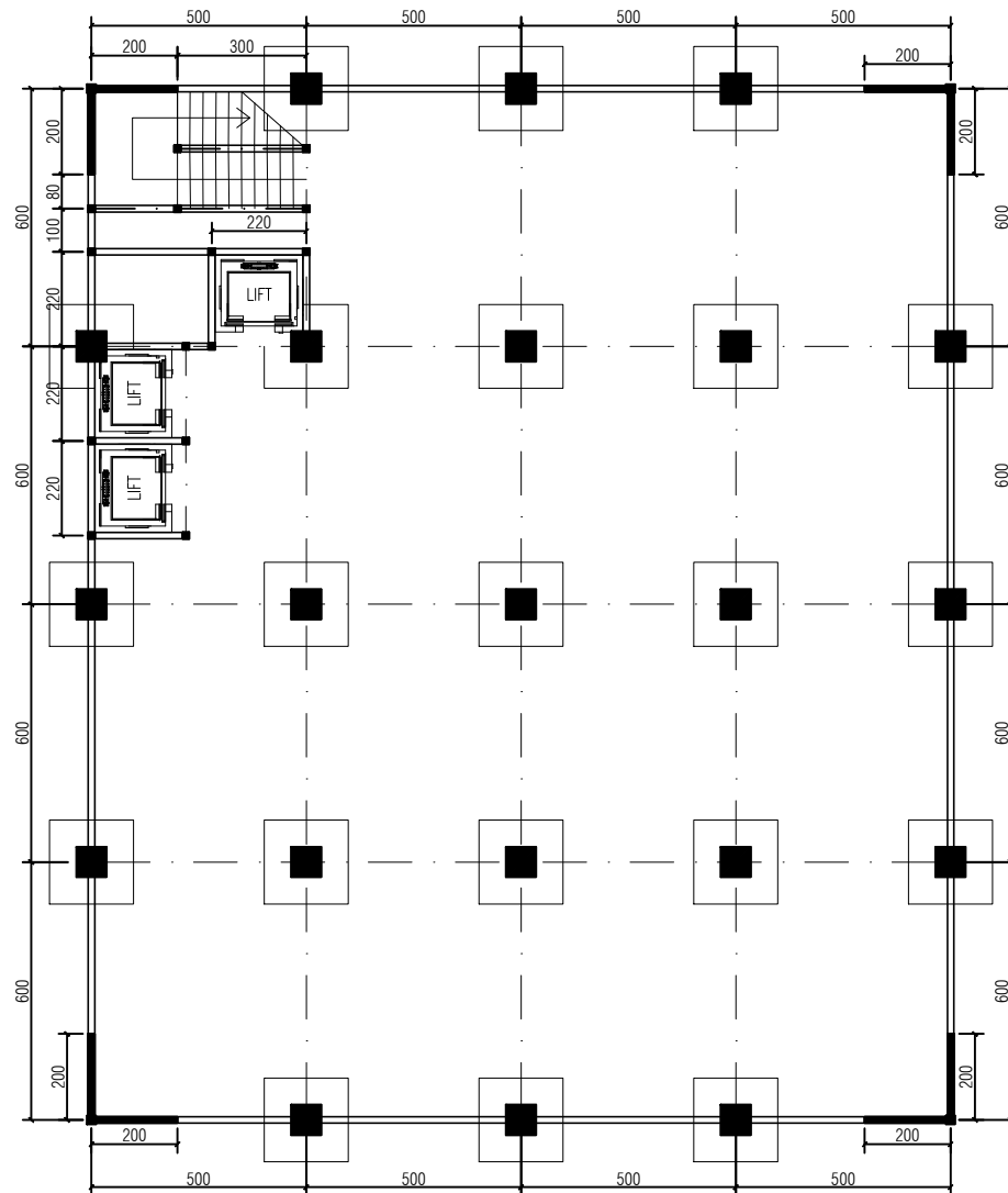
DENAH KOLOM DAN SHEARWALL SKALA 1 : 1
