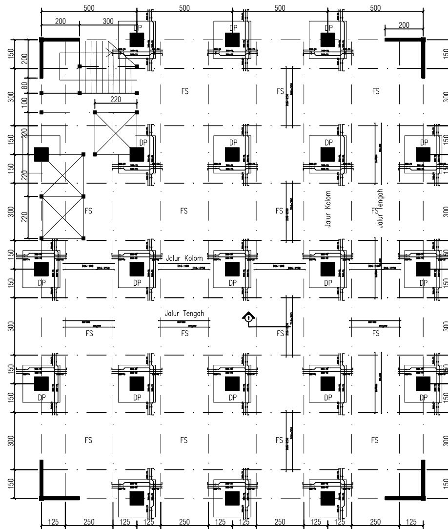
DETAIL PENULANGAN FLAT SLAB SKALA 1 : 1
