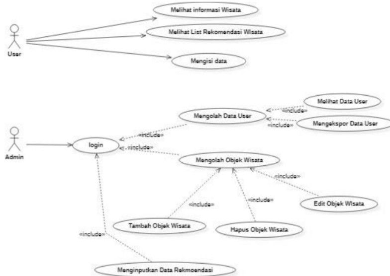
Gambar 1. Use Case Diagram Sistem Rekomendasi Wisata
