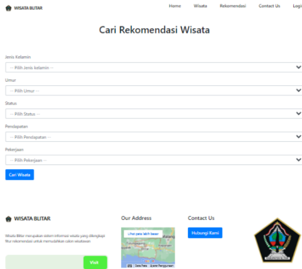
Gambar 8. Halaman Rekomendasi
