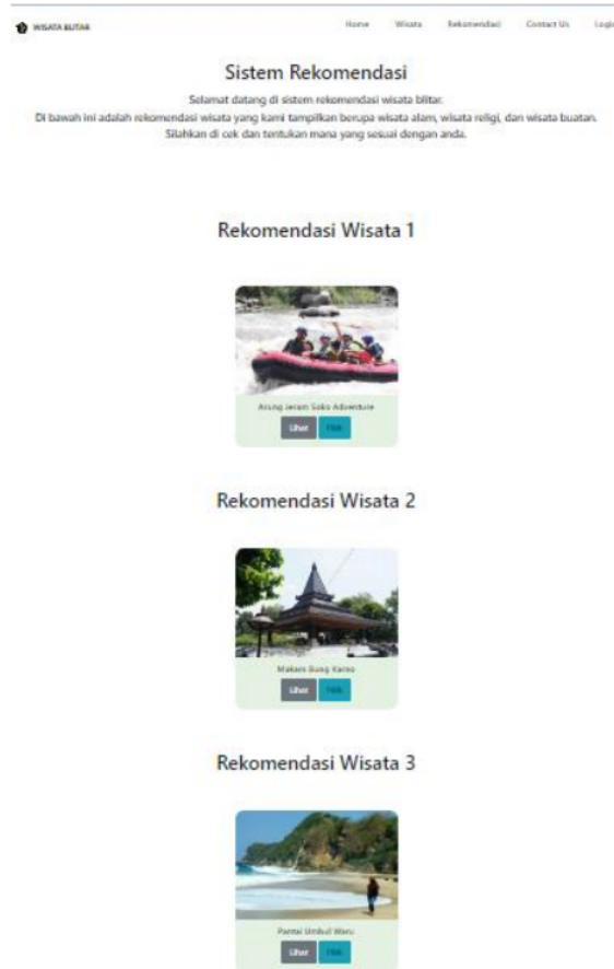
Gambar 9. Hasil rekomendasi
