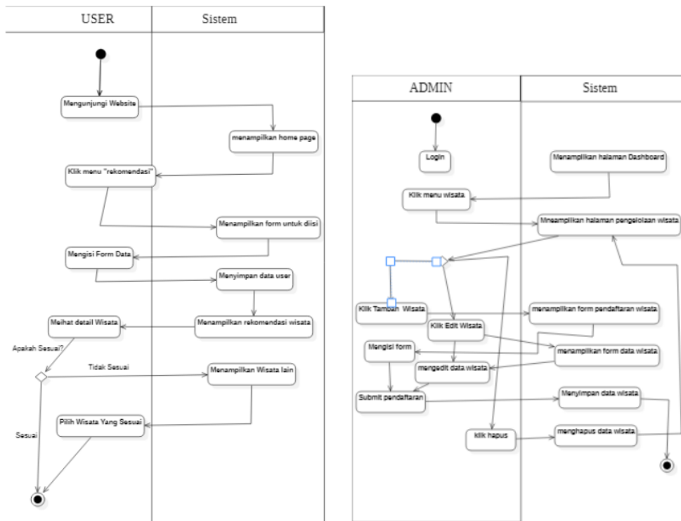
Gambar 2. Activity diagram (kiri) lihat rekomendasi (kanan) mengelola objek wisata
