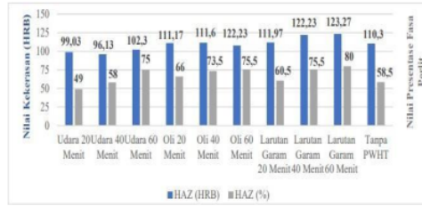
4 Gambar 14. Hubungan pengaruh variasi waktu tahan PWHT dan media pendingin terhadap kekeerasan & struktur mikro (HAZ)
