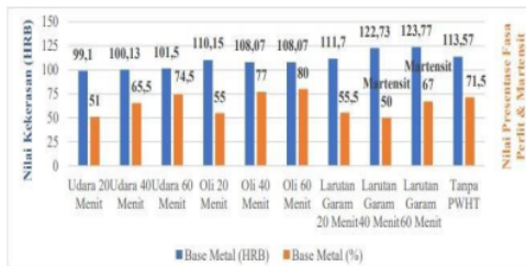
2 Gambar 13. Hubungan Pengaruh Variasi Waktu Tahan PWHT Dan Media Pendingin Terhadap Kekeerasan & Struktur Mikro (Base Metal)
