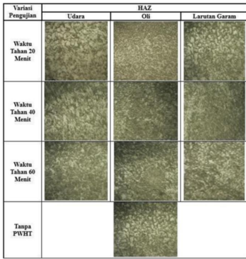
Gambar 10. Hasil uji struktur mikro daerah HAZ
