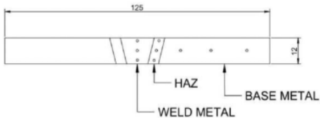
Gambar 5. Titik pengujian kekerasan Rockwell
