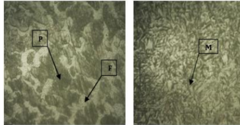
Gambar 8. Struktur mikro pada spesimen
