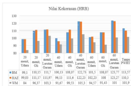
Gambar 7. Diagram nilai kekerasan pengaruh PWHT waktu tahan dan media pendingin
