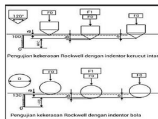
Gambar 1. Skema pengujian kekerasan rockwell .
