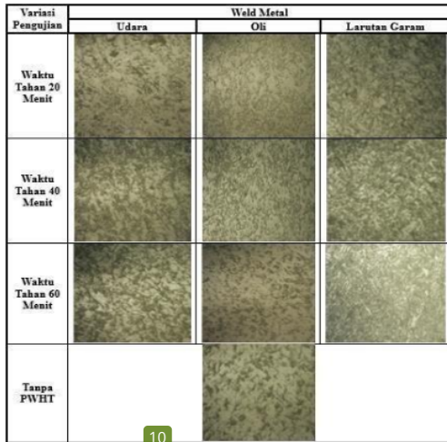
Gambar 11. Hasil uji struktur mikro daerah Weld Metal
