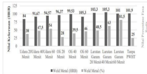
4 Gambar 15. Hubungan pengaruh variasi waktu tahan PWHT dan media pendingin terhadap kekeerasan & struktur mikro (Weld Metal)
