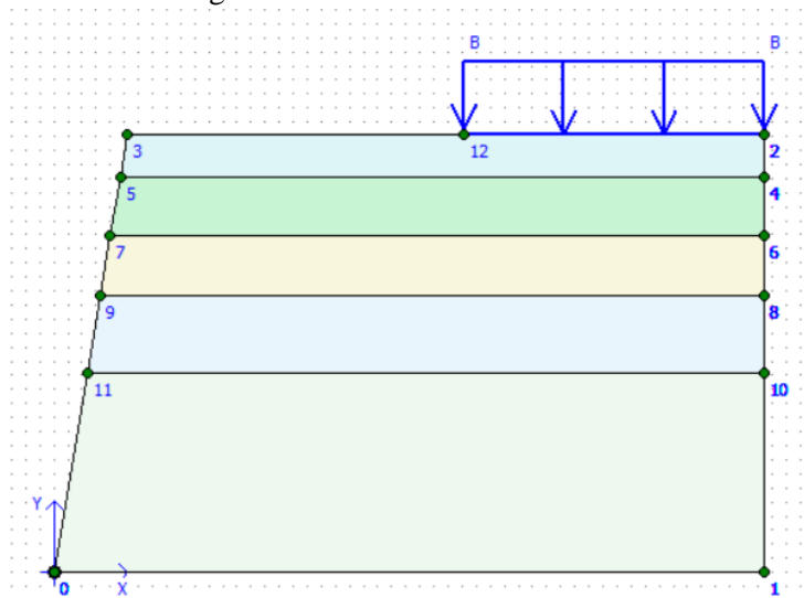
Gambar 3 Permodelan Lereng Input Plaxis
