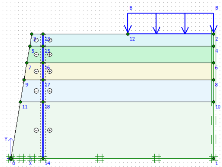
Gambar 9 Permodelan Lereng Input Plaxis
