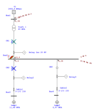
Gambar 3. Simulasi ETAP Pada Sisi Incoming
