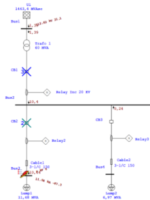
Gambar 4. Simulasi ETAP Pada Sisi Penyulang
