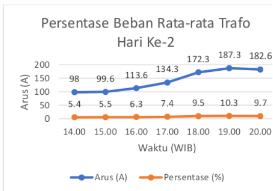
Gambar 4 Grafik Persentase Beban Rata-rata Hari Ke-2
