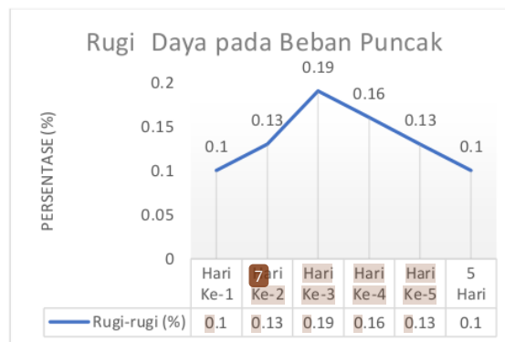
Gambar 10 Grafik Rugi-rugi Daya Pada Saat Beban Puncak
