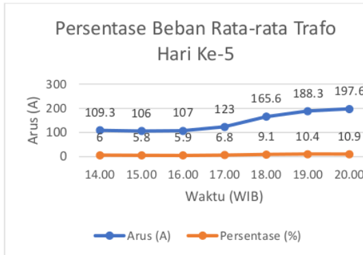
Gambar 7 Grafik Persentase Beban Rata-rata Hari Ke-5
