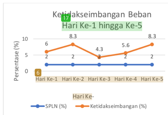
Gambar 9 Grafik Ketidakseimbangan beban pertama hingga terakhir
