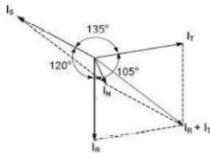
Gambar 1 Diagram Vektor Arus Keadaan Tidak Seimbang
