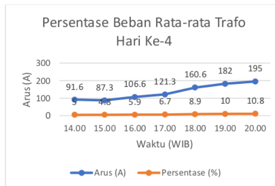
Gambar 6 Grafik Persentase Beban Rata-rata Hari Ke-4
