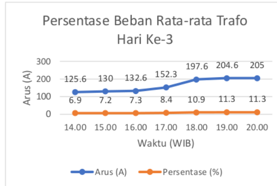
Gambar 5 Grafik Persentase Beban Rata-rata Hari Ke-3
