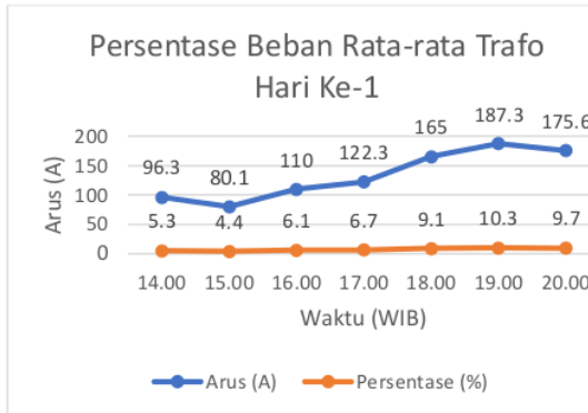
Gambar 3 Grafik Persentase Beban Rata-rata Hari Ke-1
