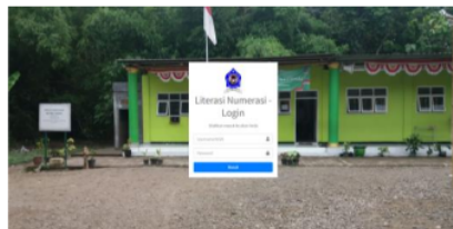
Gambar 3. Halaman Login
