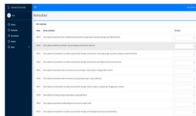
Gambar 4. Halaman Konsultasi
