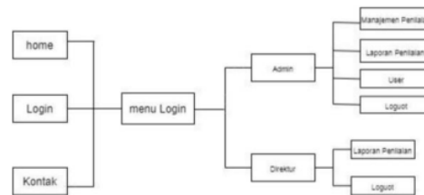
Gambar 4 Arsitektur Sitem
