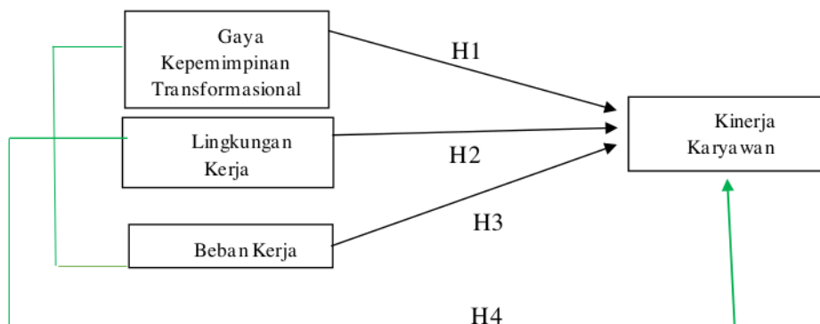
Gambar 2. 1 Kerangka Konseptual
