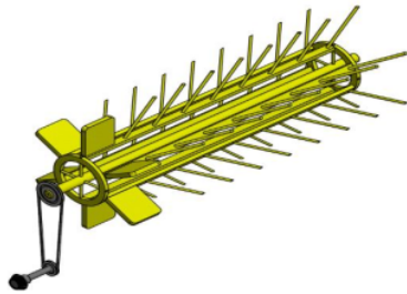
Gambar output penggerak V-Belt penggiling
