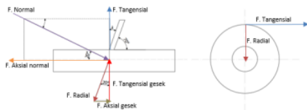
Gambar Gaya-Gaya Pada Silinder Perontok
