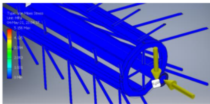
Gambar Hasil Ansys Silinder Perontok Pada Software
