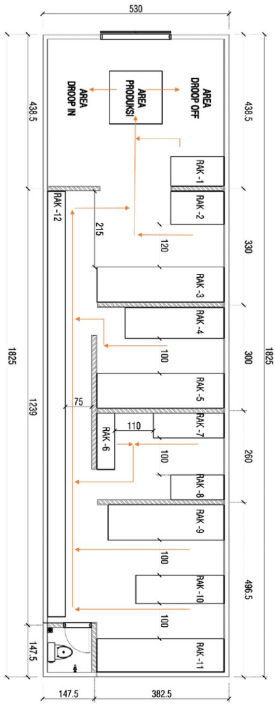
Gambar 4. Pola Alur Barang
