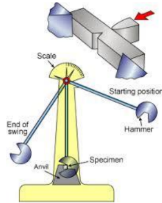
Gambar 6 uji impak
