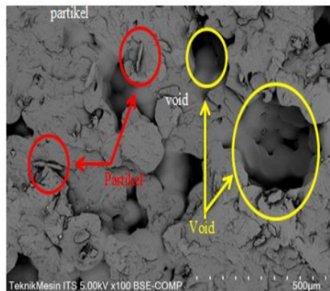
Gambar 12 20 rpm, dan 10 menit (2)
