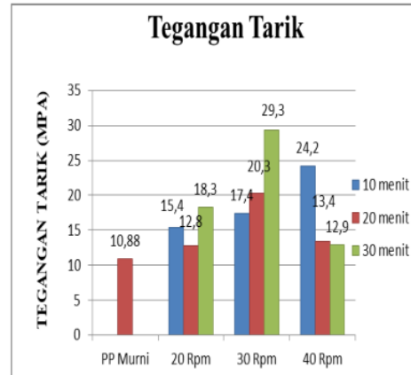
Gambar 8 Grafik tegangan tarik antara kecepatan
