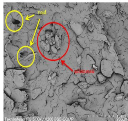
Gambar 10 SEM 40 rpm, dan lama pengadukan 10 menit
