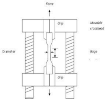
Gambar 5 pengujian Tarik
