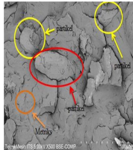
Gambar 9 SEM 40 rpm, dengan lama pengadukan 10 menit
