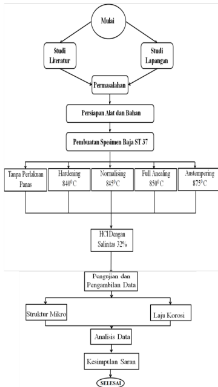
Gambar 1. Skema pengujian perlakuan panas
