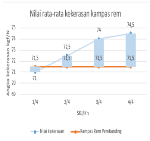
Gambar 9 Grafik Hasil pengujian kekerasan variasi SKJ/Kuningan
