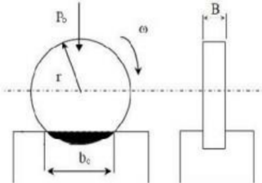
Gambar 7 Ilustrasi Pengujian Ogoshi
