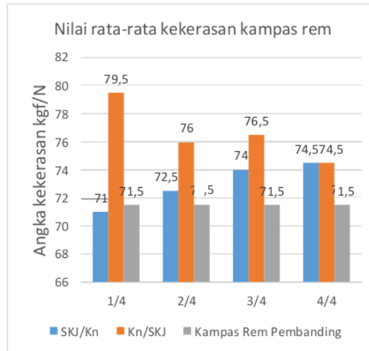
Gambar 10 Grafik Hasil pengujian kekerasan kombinasi
