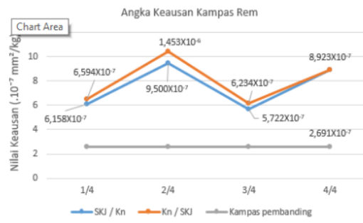
Gambar 13 grafik kombinasi
