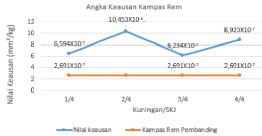
Gambar 12 Grafik keausan kampas rem variasi kuningan/serbuk kayu jati
